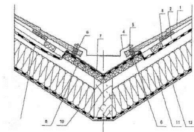
Рис. 14. Ендова кровли
