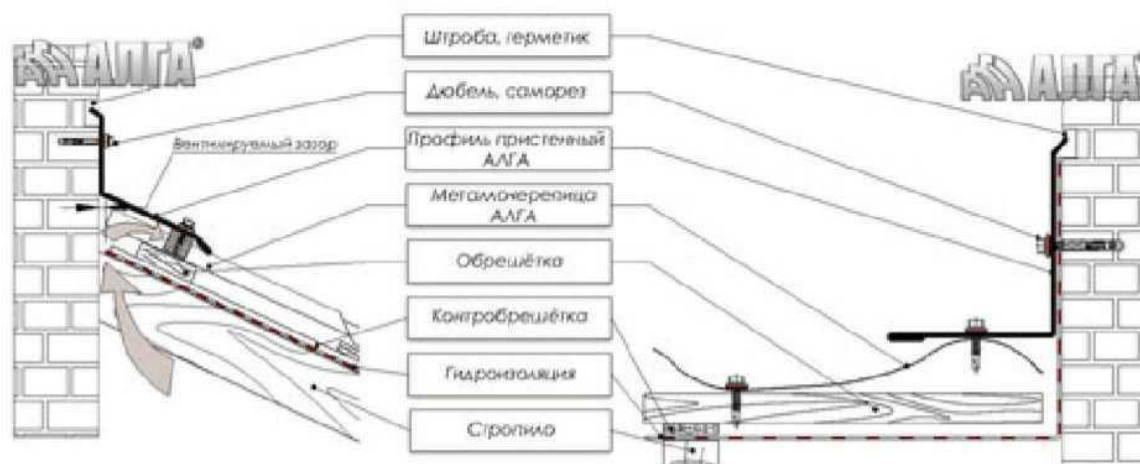
Рис. 17. Пристенный узел
